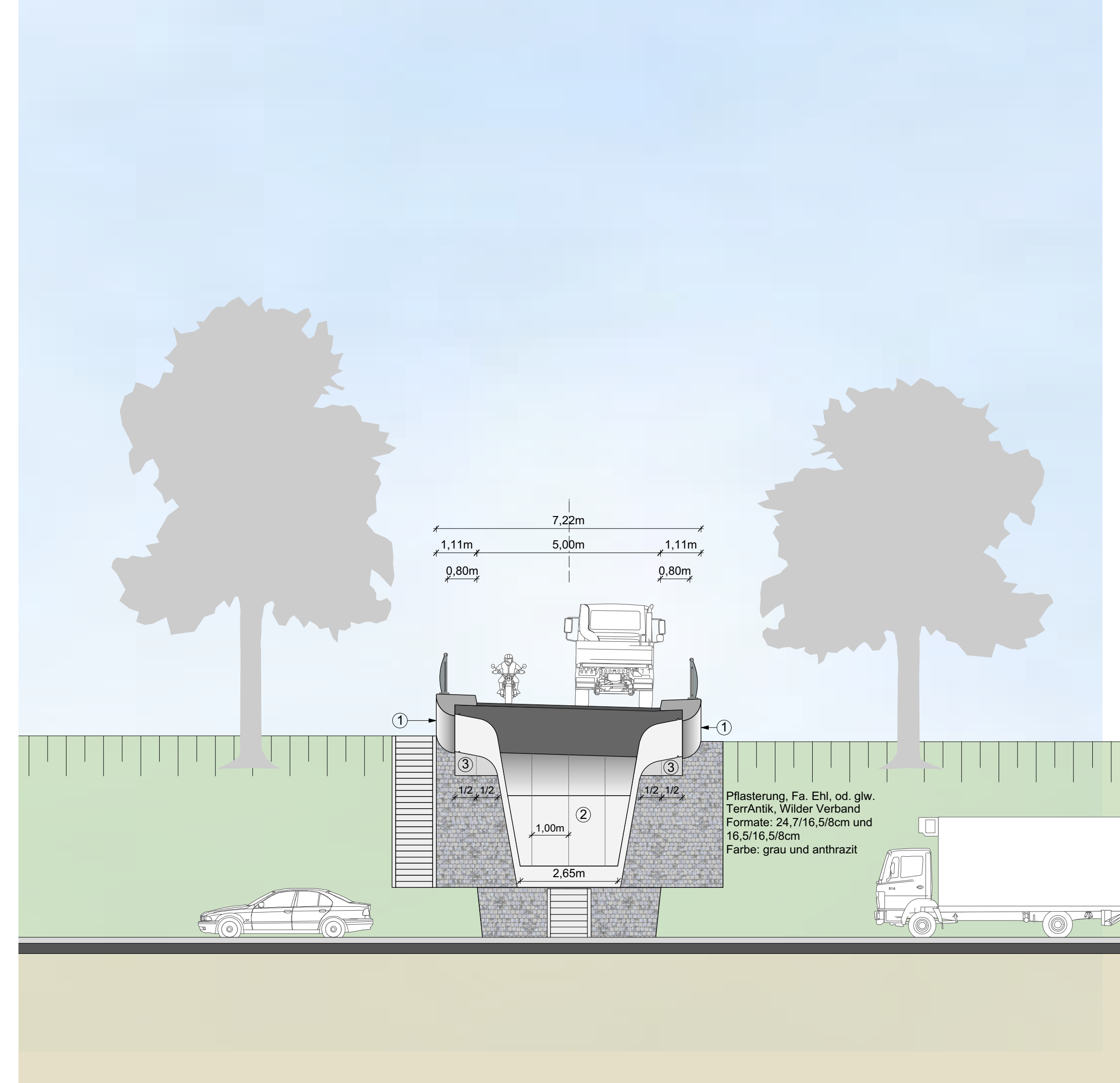
Anzicht Widerlager Ost
