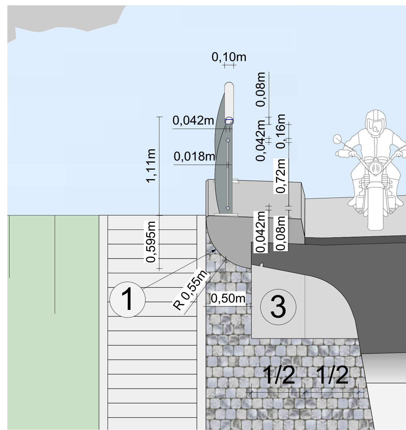
Ausschnitt Geländer M. 1 : 25
