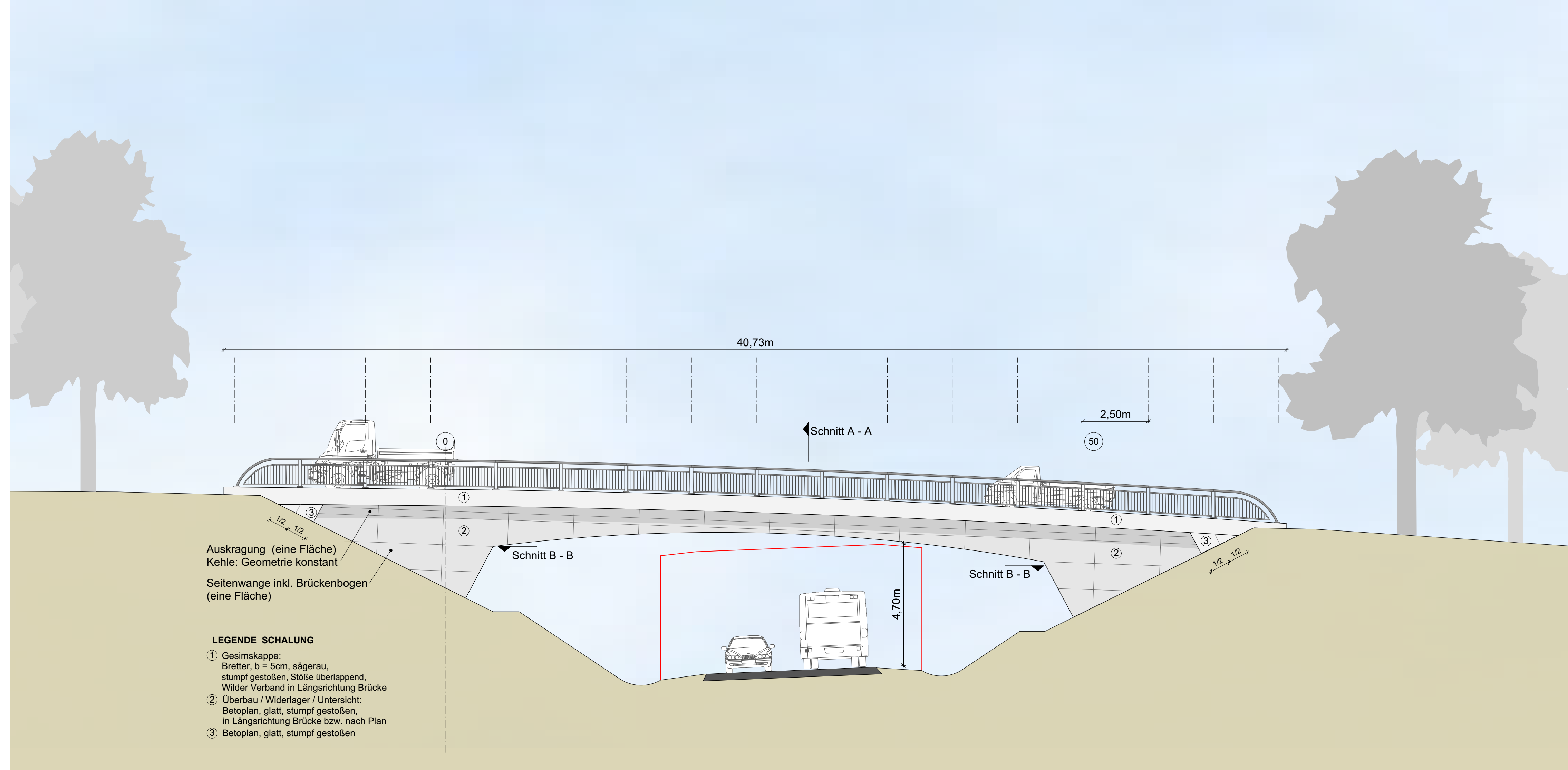
Anzicht von Norden
