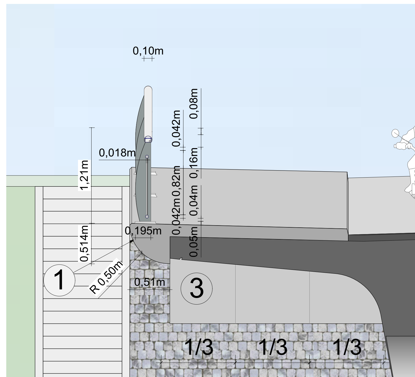
Ausschnitt Geländer M. 1 : 25
