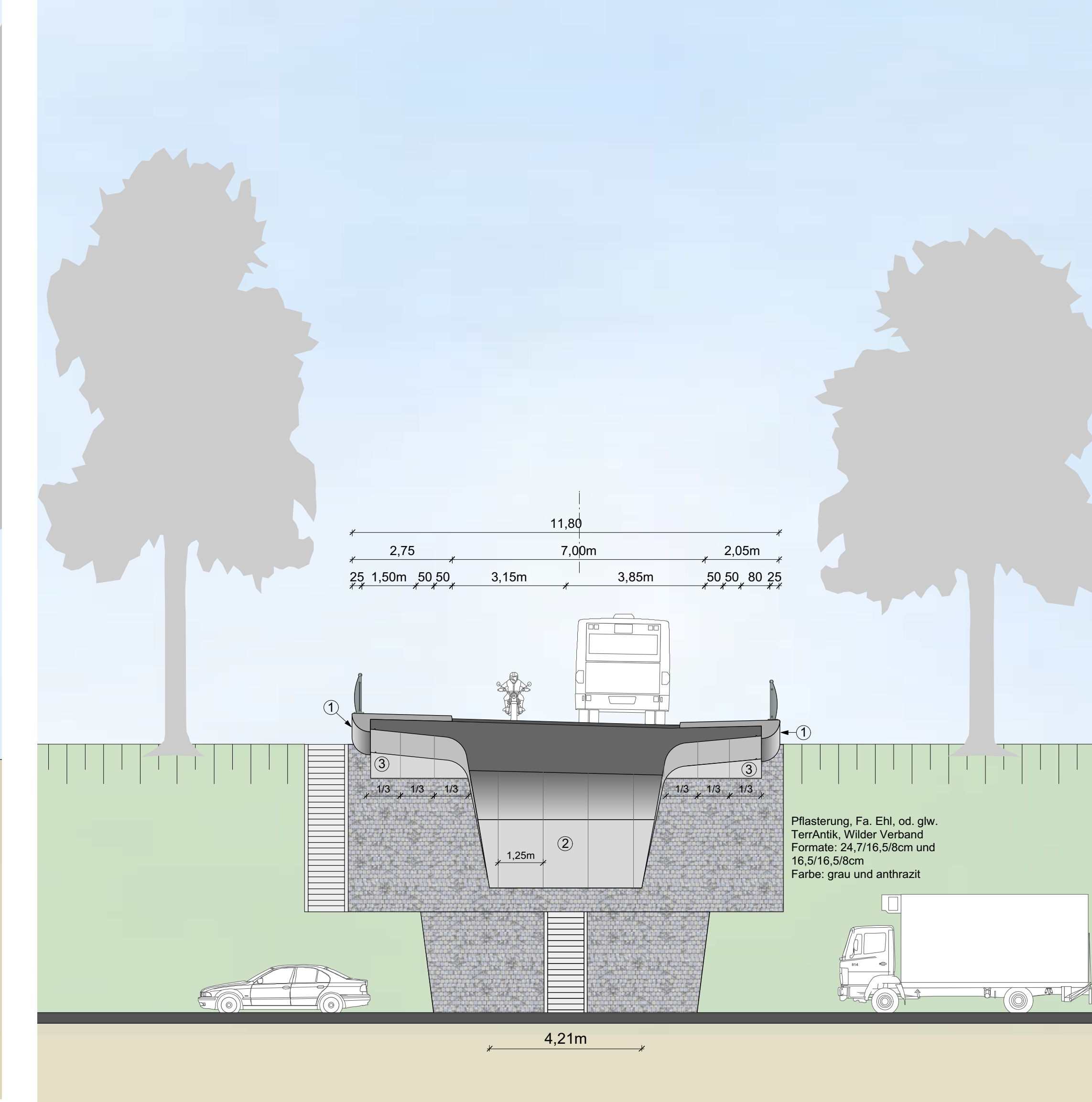
Ansicht Widerlager Ost
