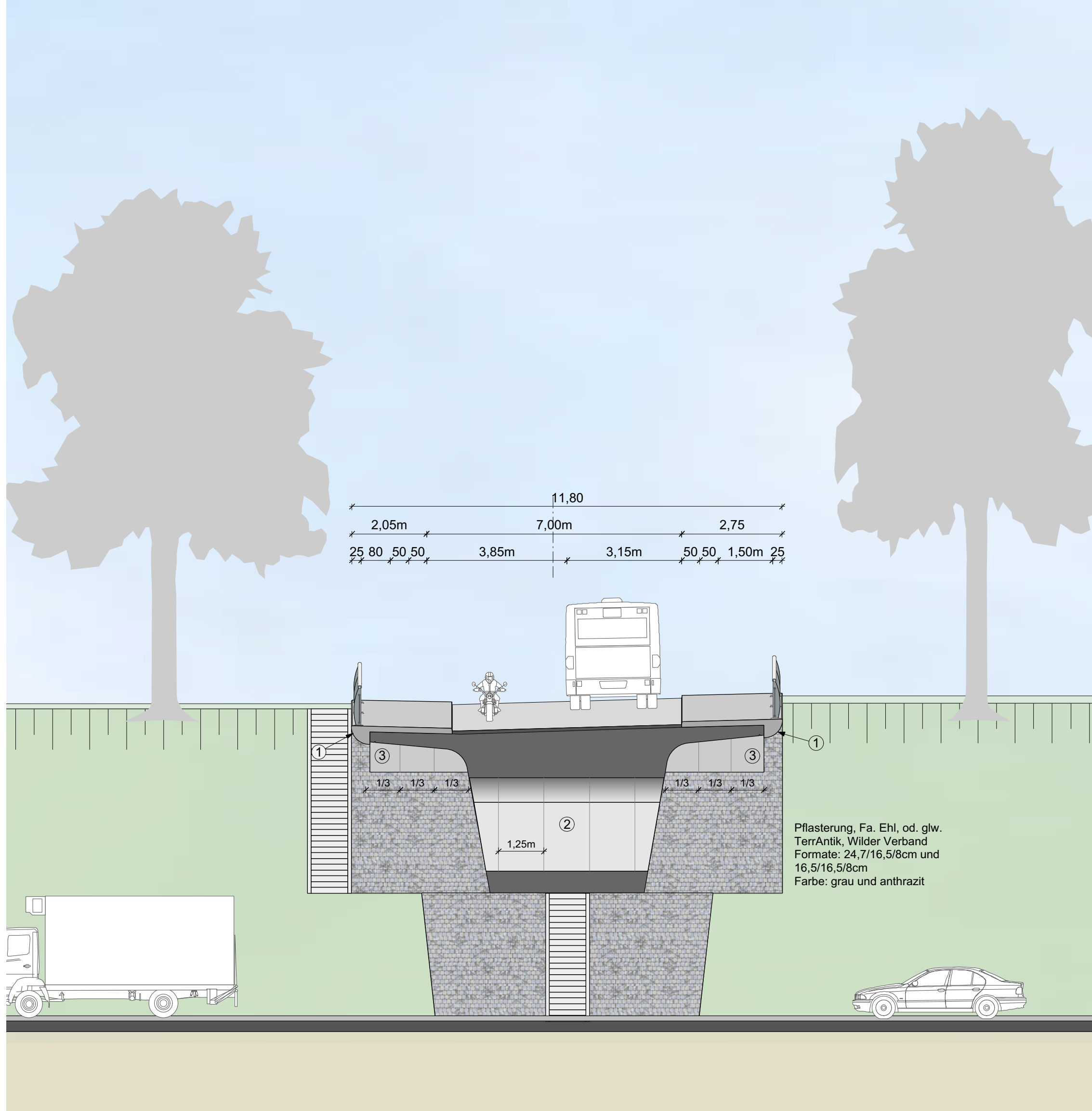
Ansicht Widerlager West Schnitt A - A
