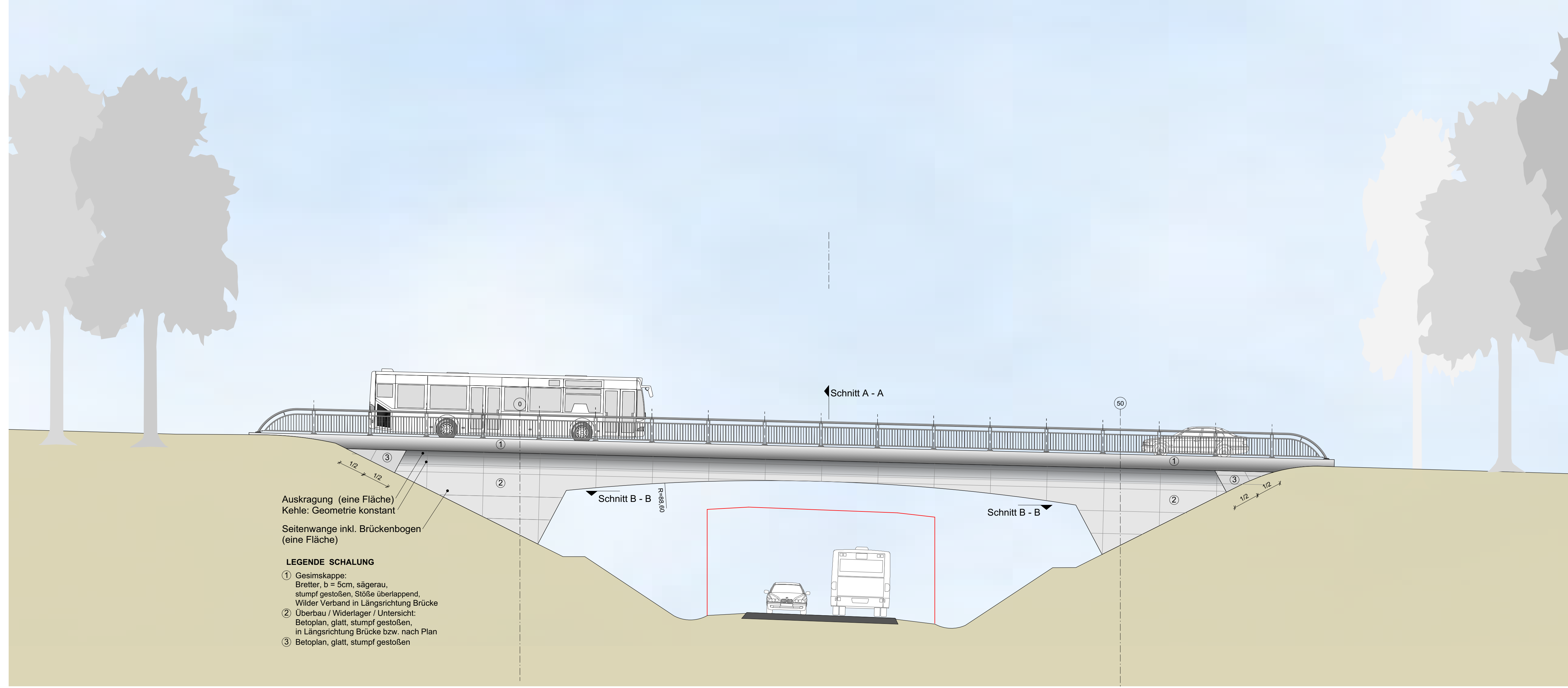
Ansicht von Norden Ansicht / Schnitt 2 - 2
